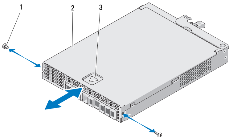
图 16-9. 打开和关闭 RAID 控制器模块
